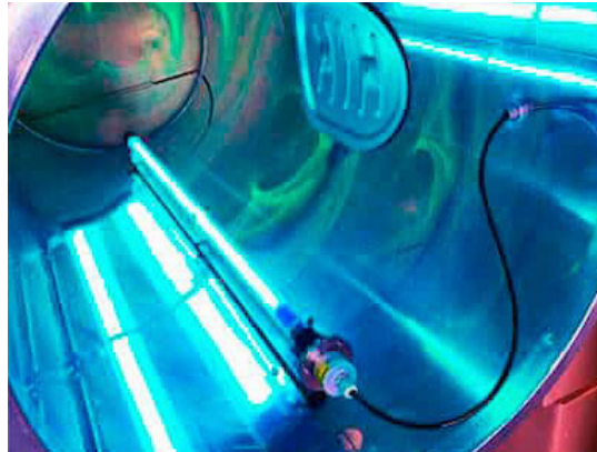
Instal·lació de generadors d'UV-C en els conductes; si cal s'instal·len tapes de registre per facilitar el muntatge i el manteniment.
